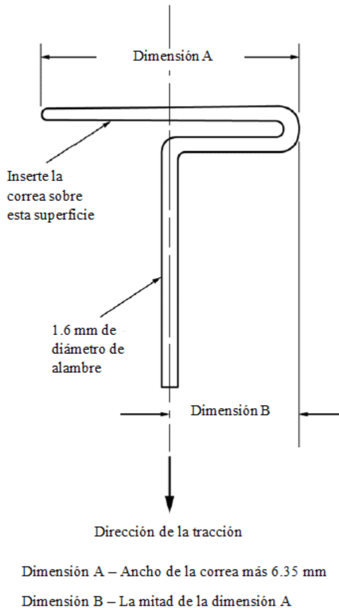
Figura 3-Dispositivo de tracción
