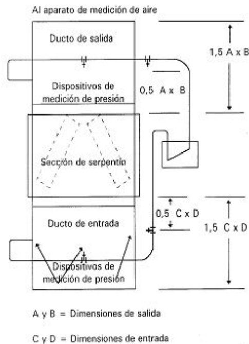
FIGURA 8. Medición de caída de presión estática del aire para una sección de serpentín sin ventiladores
