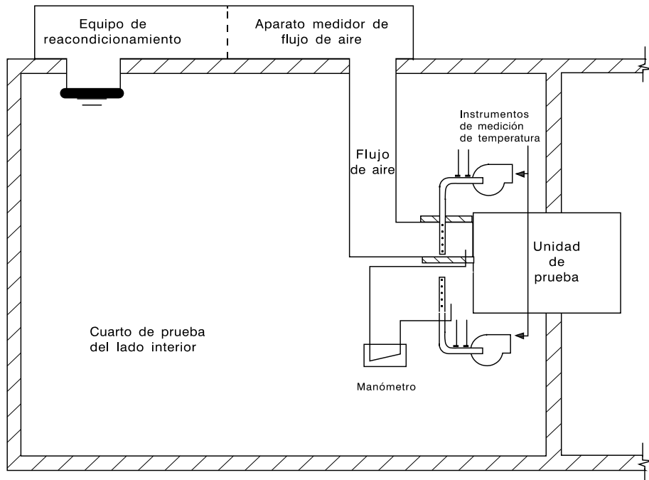
FIGURA 4. Cuarto de aire - entalpía
